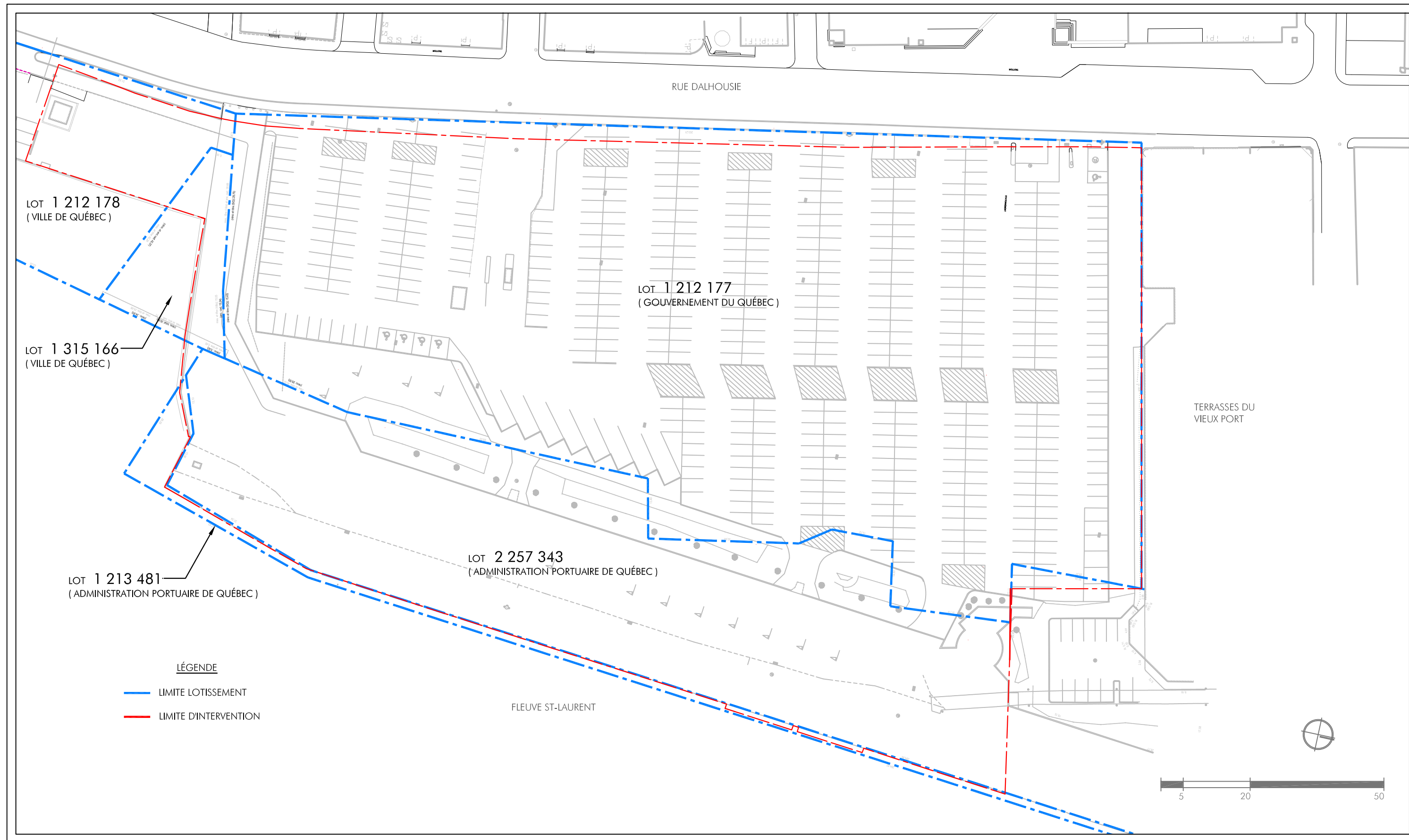
PLACE DES CANOTIERS PLAN 1: SITUATION ACTUELLE, LOTISSEMENT ET LIMITE D'INTERVENTION
