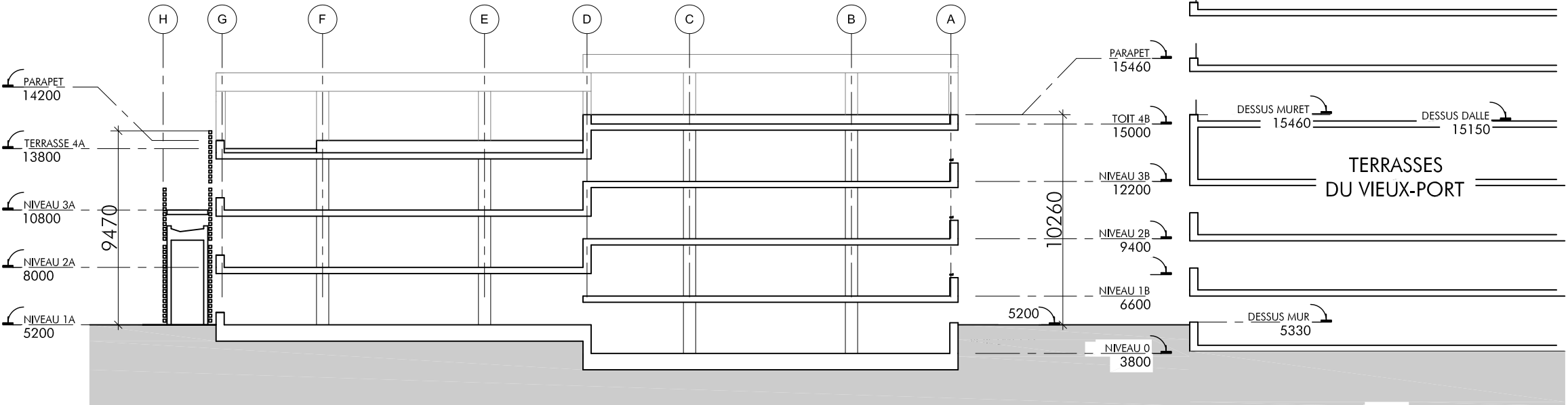
COUPE 1
