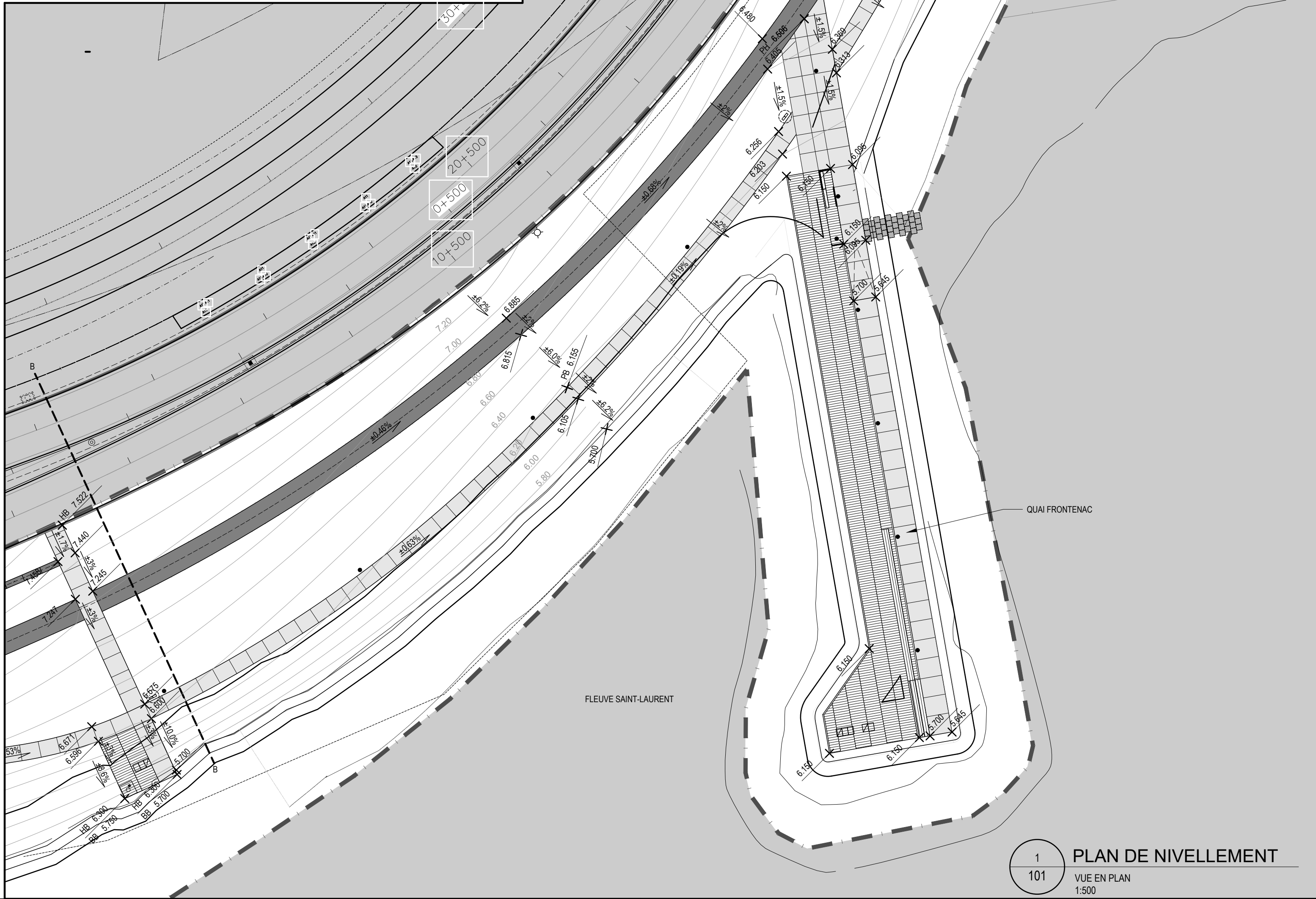
2 101 PLAN DE NIVELLEMENT VUE EN PLAN 1:500
