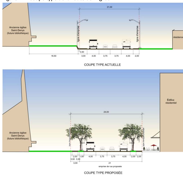
Figure 42 : Coupe type de la route de l'Église
